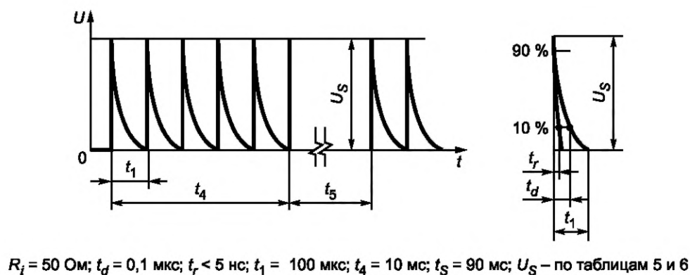
Рисунок 17 — Форма и параметры испытательных импульсов 3б
