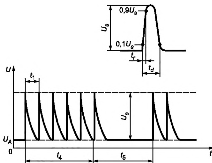
Рисунок 9 — Испытательный импульс 3b
