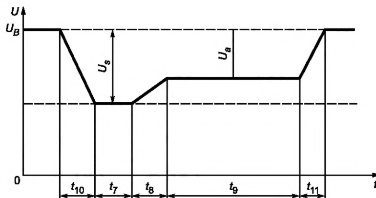
Рисунок 10 — Испытательный импульс 4
