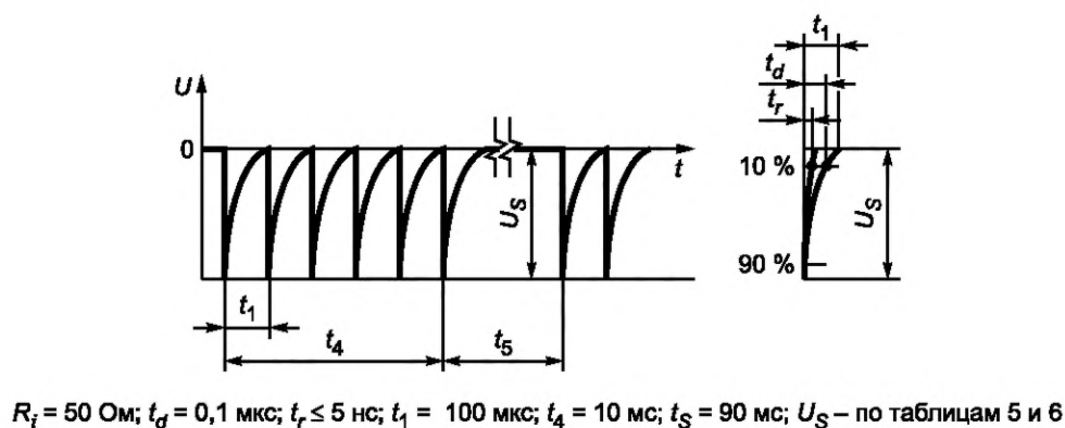
Рисунок 16 — Форма и параметры испытательных импульсов 3а
