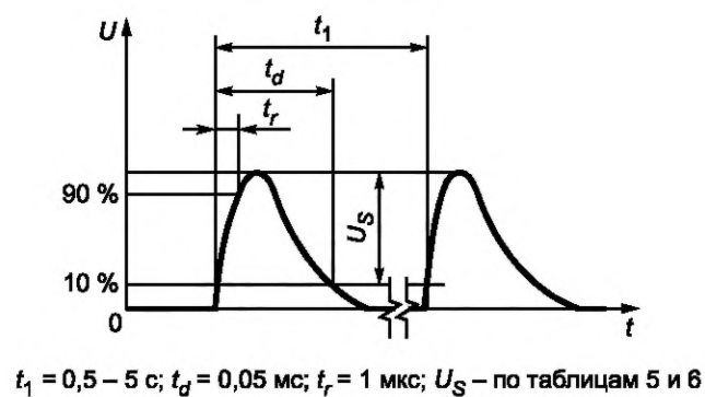
Рисунок 15 — Форма и параметры испытательного импульса 2
